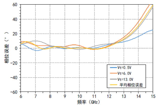
相位误差VS频率@Pin=-10dBm
