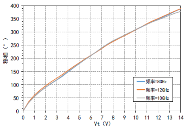
移相VS Vt@Pin=-10dBm
