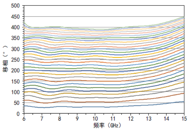
移相VS频率@Pin=-10dBm (Vt=0.5V~15V)
